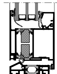
Lodret snit indadgående dør
