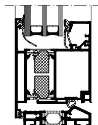
Lodret snit udadgående dør
