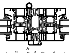
Vandret snit: Folde-/drejeelement
