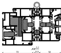
Vandret snit: Karm mod væg
