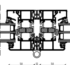
Vandret snit: Foldedør
