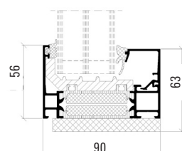
Profil mål, fast felt
