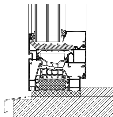
Tilslutningsprincip, oplukkeligt vindue
