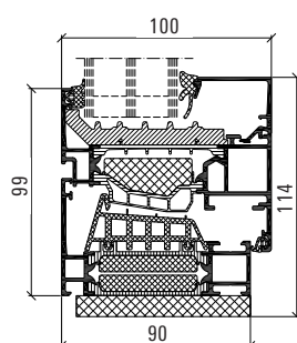
Profil mål, oplukkeligt vindue
